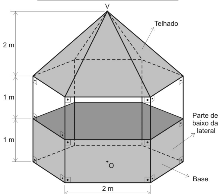
MODELO DA BARRACA PADRÃO
